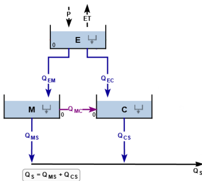
Slika 3.2 Struktura modela izvora Opačac
