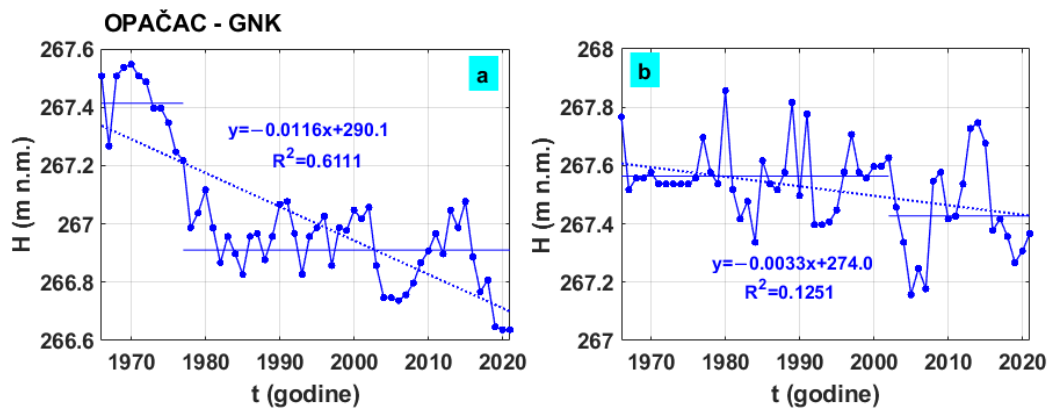
Slika 2.21 Prikaz kretanja (a) srednjih i (b) maksimalnih vodostaja na hidrološkoj postaji Opačac – Glavni natapni kanal
