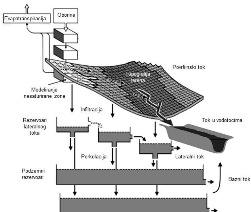
Slika 3.12 Struktura modela s primjenom metode linearnog rezervoara (modificirano prema Graham & Butts (2005) )
