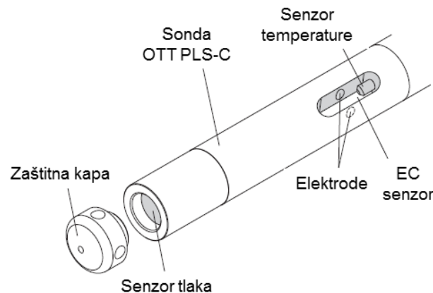
Slika 2.3 Građa višeparametarske sonde OTT PLS-C (Izvor: Operating instructions, Pressure Probe with Conductivity Sensor OTT PLS-C)
