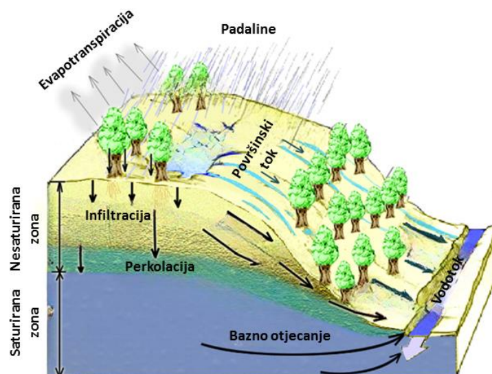
Slika 3.6 Modelirani hidrološki procesi u MIKE SHE-u (modificirano prema Tarboton, (2003))
