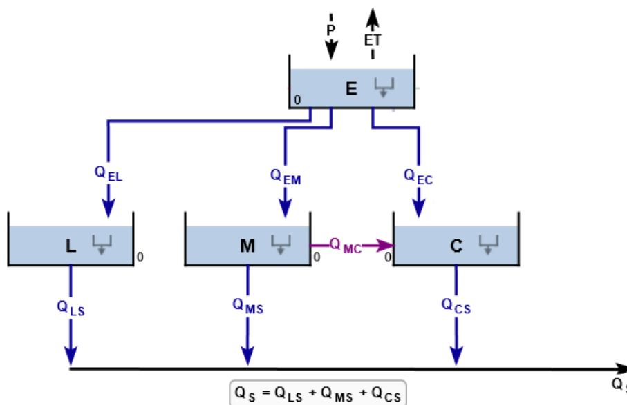
Slika 3.4 Struktura modela izvora Opačac s odjeljkom L koje simulira Crveno jezero
