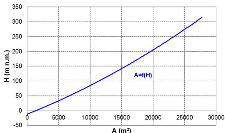
Slika 3.9 Krivulja promjene površine jezera u funkciji razine vode
