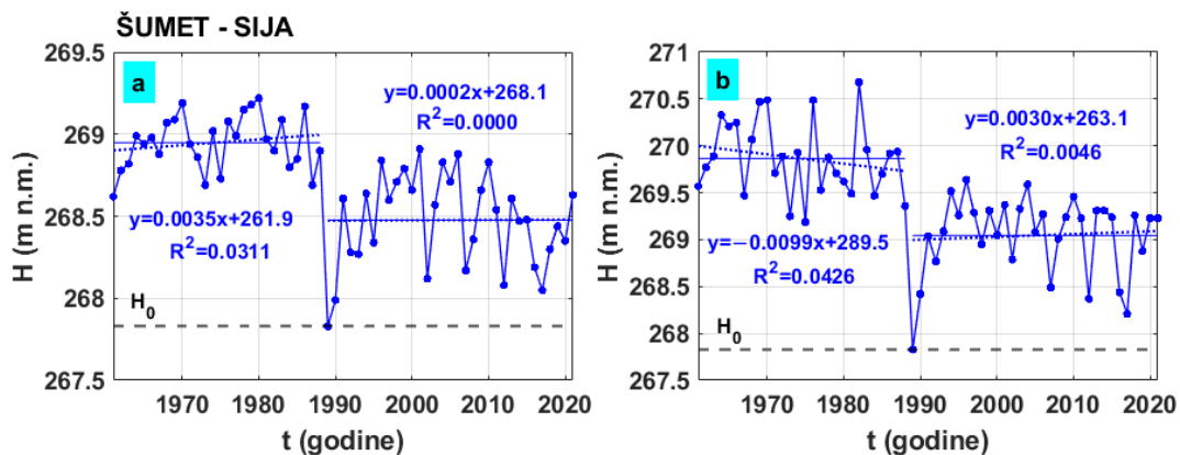
Slika 2.17 Prikaz kretanja (a) srednjih i (b) maksimalnih vodostaja na hidrološkoj postaji Šumet – Sija; H_0 = kota nule vodokaza od 267.829 m n.m.
