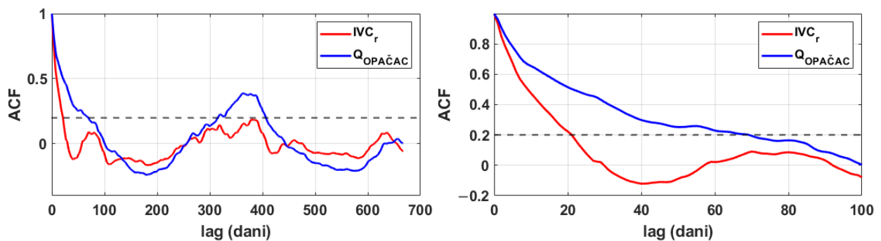
Slika 2.29 Autokorelacijska funkcija integralnih promjena volumena u Crvenom jezeru i protoka na Opačcu
