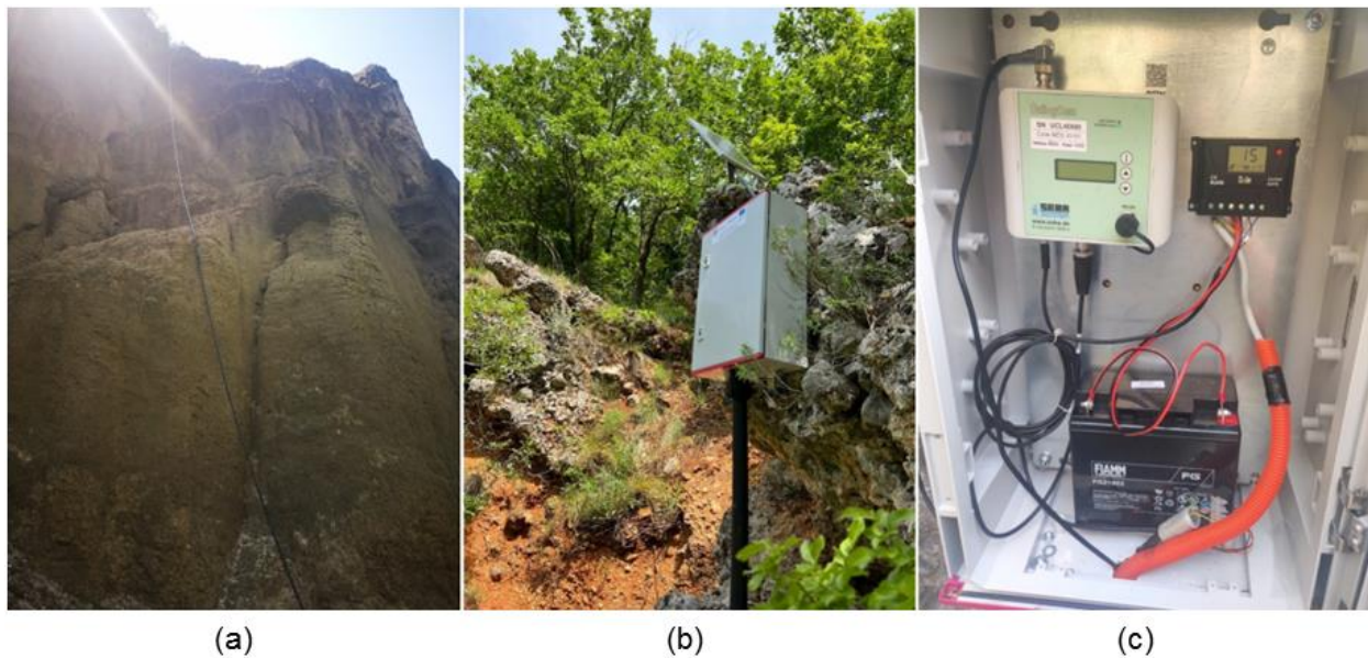
Slika 2.2. Instalacija mjernih postaja: (a) spuštanje kabela u Modrom jezeru, (b) dojavna stanica sa solarnim panelom u jezeru Galipovac, (c) unutrašnjost dojavne stanice instalirane u Crvenom jezeru
