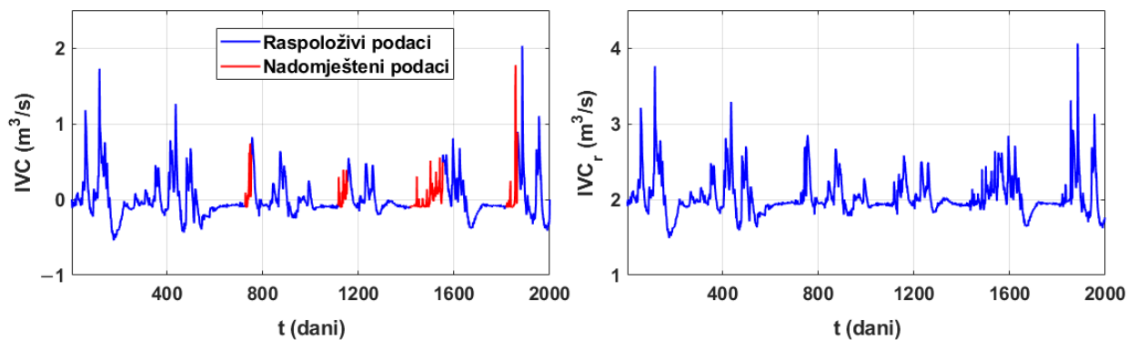
Slika 2.26 Integralne promjene volumena Crvenog jezera s imputiranim nedostajućim vrijednostima i transformirane vrijednosti integralnih promjena volumena IVC_r
