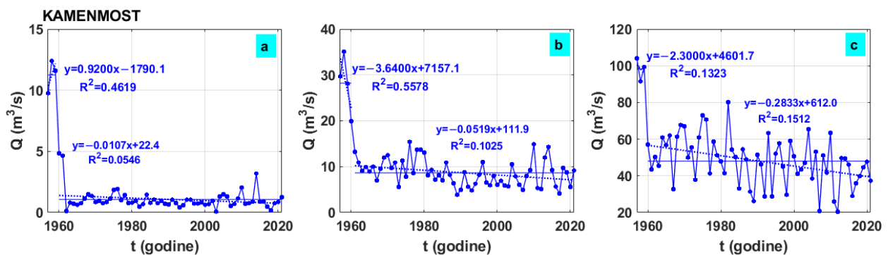
Slika 2.24 Prikaz kretanja (a) minimalnih, (b) srednjih i (c) maksimalnih godišnjih protoka na hidrološkoj postaji Kamenmost
