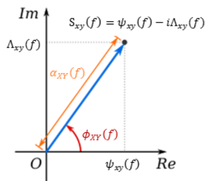
Slika 1.8 Trigonometrijski prikaz kompleksnog broja u pravokutnom koordinatnom sustavu
