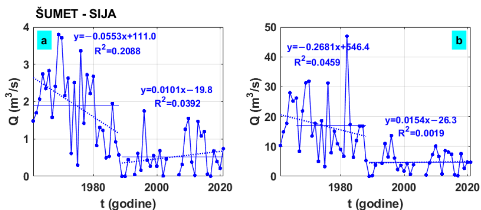
Slika 2.18 Prikaz kretanja (a) srednjih i (b) maksimalnih protoka na hidrološkoj postaji Šumet – Sija
