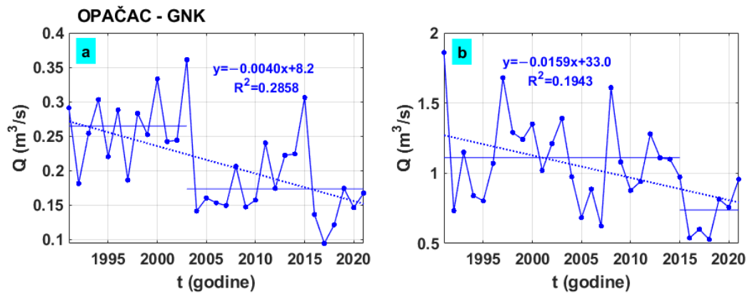
Slika 2.22 Prikaz kretanja (a) srednjih i (b) maksimalnih protoka na hidrološkoj postaji Opačac – Glavni natapni kanal
