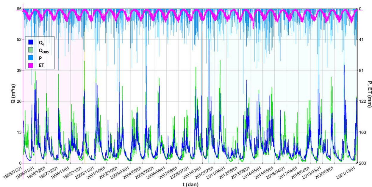
Slika 3.3 Usporedba hidrograma mjenjenih vrijednosti protoka i simuliranih vrijednosti protoka na izvoru Opačac uz prikaz vremenske serije ulaznih podataka oborina i referentne evapotranspiracije
