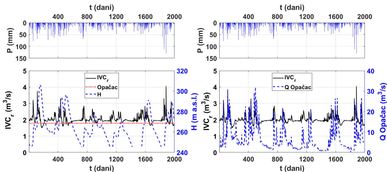
Slika 2.27 Usporedba padalina na mjernoj postaji Imotski s integralnim promjenama volumena u Crvenom jezeru ( IVC_r ), razinama u jezeru ( H ) i protocima na izvoru Opačac
