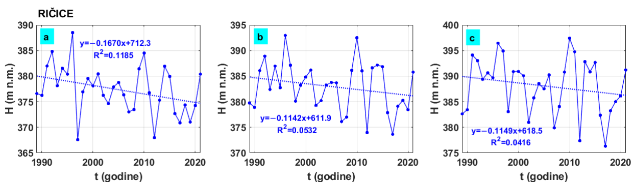
Slika 2.15 Prikaz kretanja (a) minimalnih, (b) srednjih i (c) maksimalnih vodostaja na hidrološkoj postaji Ričice
