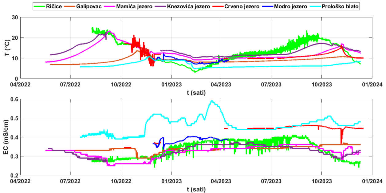
Slika 2.35 Prikaz kretanja temperature vode (T) i električne vodljivosti (EC) u jezerima za raspoložive nizove podataka
