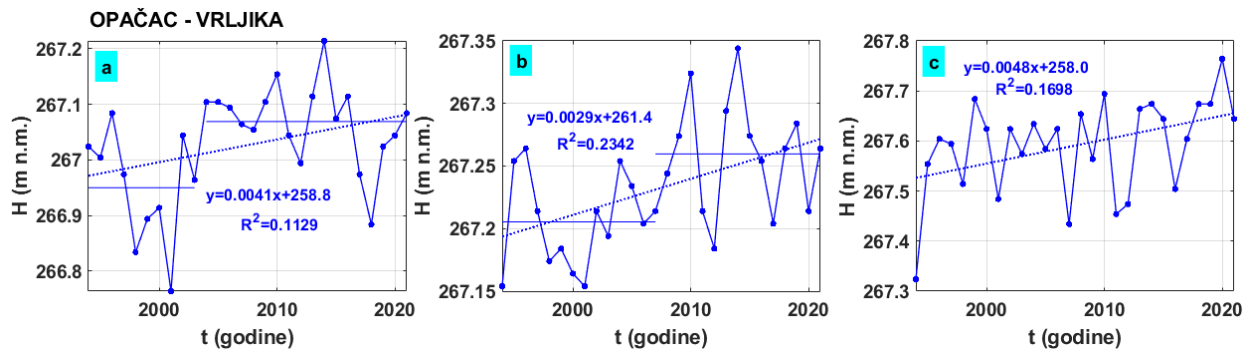
Slika 2.19 Prikaz kretanja (a) minimalnih, (b) srednjih i (c) maksimalnih vodostaja na hidrološkoj postaji Opačac – Vrljika
