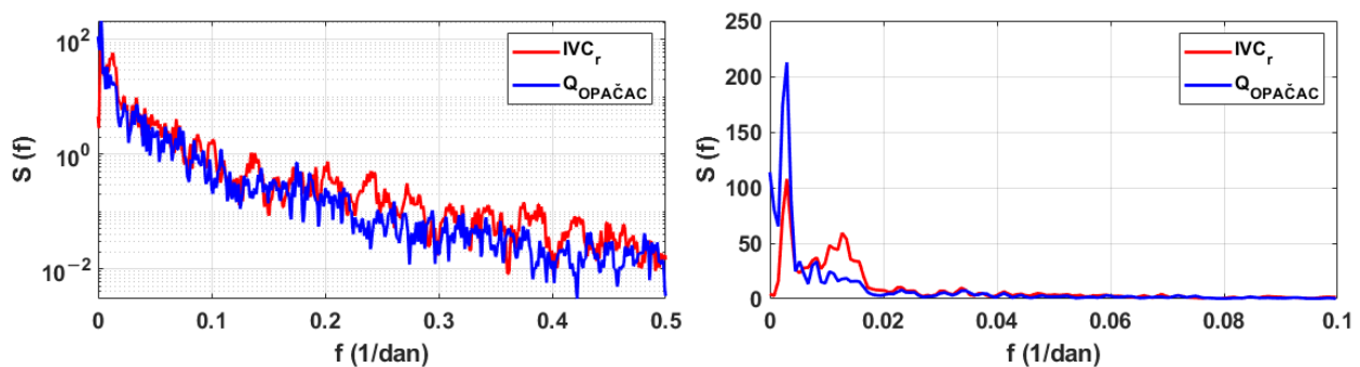
Slika 2.31 Prikaz spektralne funkcije gustoće S(f) integralnih promjena volumena te protoka na Opačcu na logaritamskom i linearnom mjerilu
