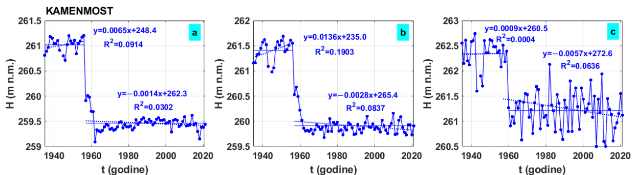
Slika 2.23 Prikaz kretanja (a) minimalnih, (b) srednjih i (c) maksimalnih vodostaja na hidrološkoj postaji Kamenmost
