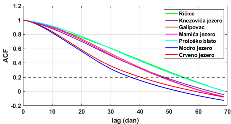
Slika 2.36 Autokorelacijske funkcije razina vode u jezerima
