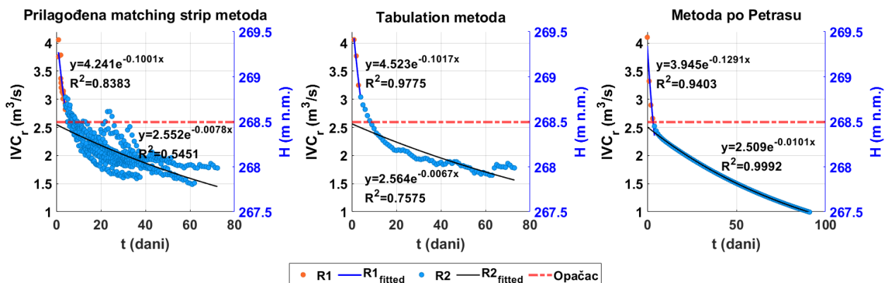
Slika 2.28 Glavna recesijska krivulja dobivena korištenjem Prilagođene matching strip metode, Tabulation metode i metode po Petrasu
