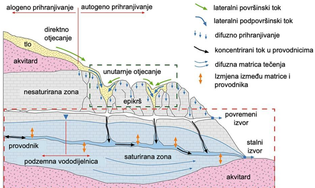
Slika 1.2 Konceptualni model krškog vodonosnika (Hartmann i ostali, 2014)
