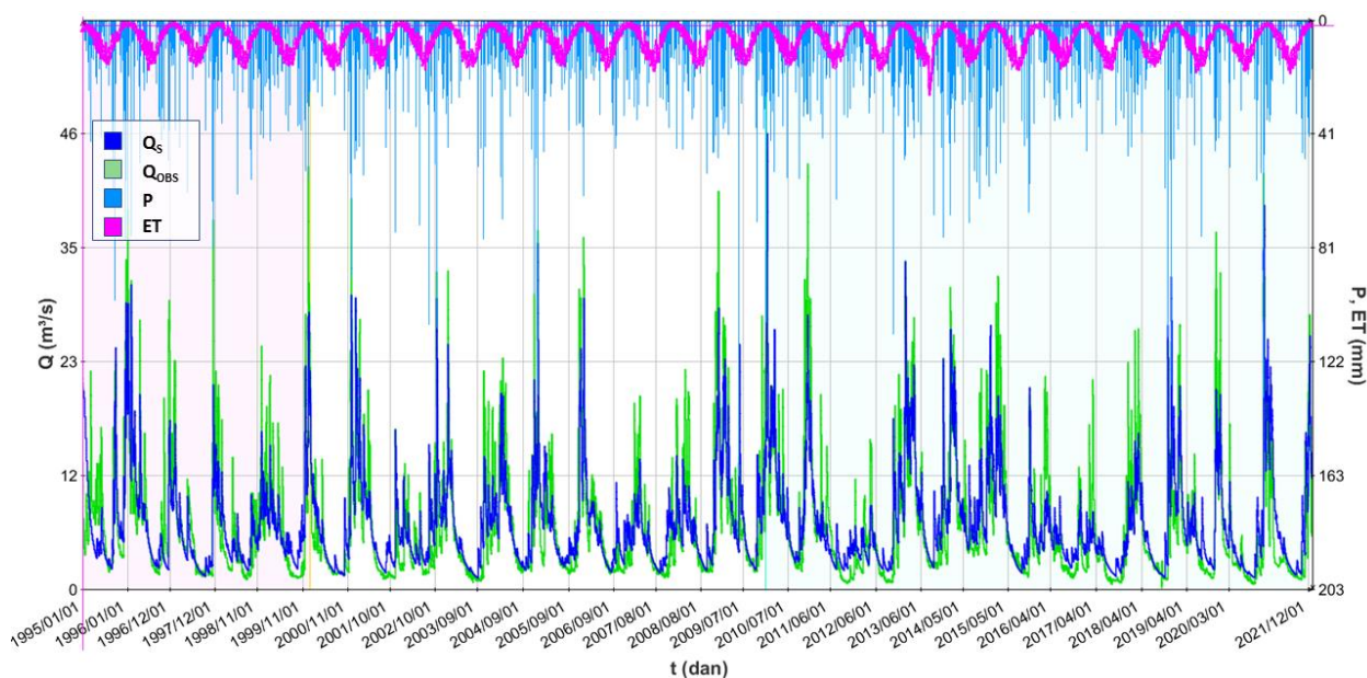
Slika 3.5 Usporedba hidrograma mjerenih vrijednosti protoka i simuliranih vrijednosti protoka na izvoru Opačac za model s Crvenim jezerom, uz prikaz vremenske serije ulaznih podataka oborina i referentne evapotranspiracije
