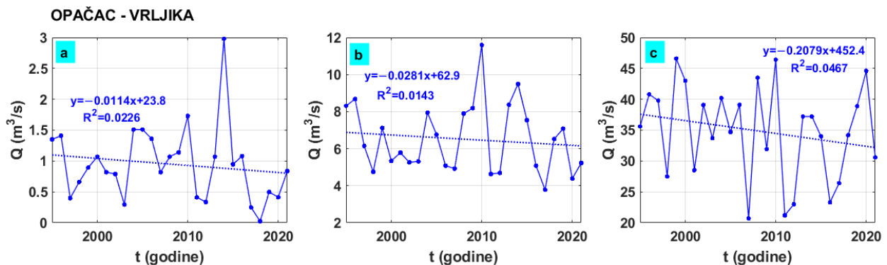
Slika 2.20 Prikaz kretanja (a) minimalnih, (b) srednjih i (c) maksimalnih godišnjih protoka na hidrološkoj postaji Opačac – Vrljika
