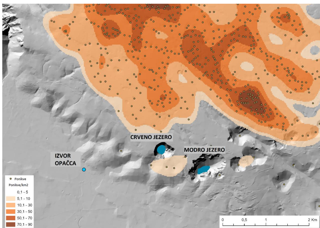
Slika 1.4 Karta gustoće ponikava (broj ponikava po km 2 ) za područje sjeveroistočno od grada Imotskog (Vrsalović i ostali, 2022)
