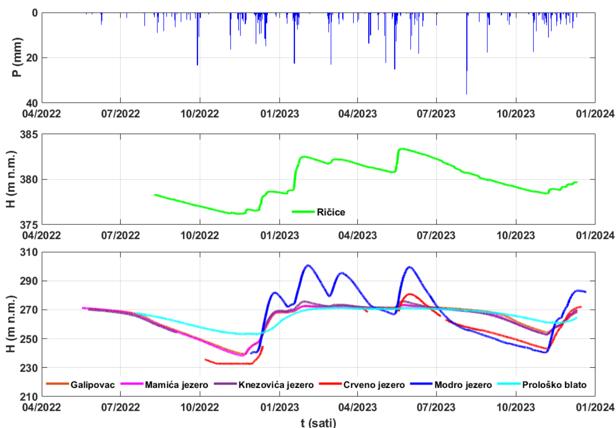
Slika 2.33. Prikaz kretanja razina vode u Ričicama, Galipovcu, Mamića jezeru, Knezovića jezeru, Crvenom i Modrom jezeru i u Prološkom blatu uz hijetogram s meteorološke postaje Runovići
