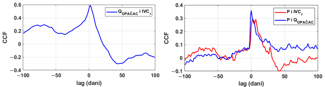
Slika 2.30 Kros-korelacijska funkcija protoka na Opačcu i integralnih promjena volumena u Crvenom jezeru ( IVC_r ) te kros-korelacijska funkcija protoka na Opačcu i integralnih promjena volumena Crvenog jezera u kombinaciji s količinom oborina s mjerne postaje Imotski
