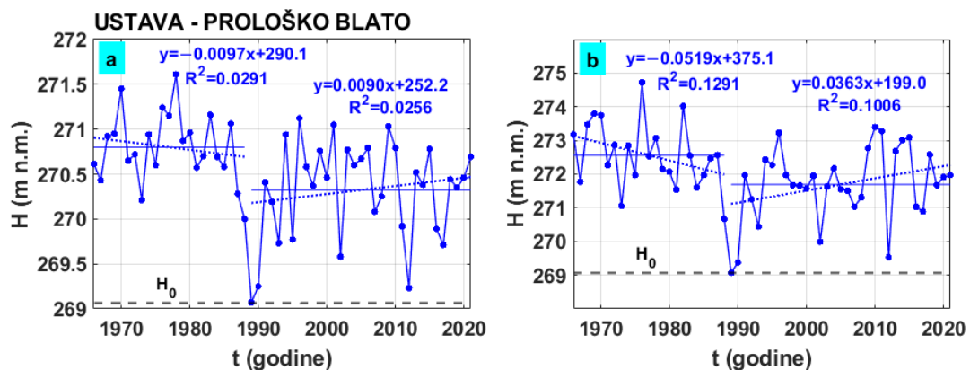
Slika 2.16 Prikaz kretanja (a) srednjih i (b) maksimalnih vodostaja na hidrološkoj postaji Ustava – Prološko blato; H_0 = kota nule vodokaza od 269.071 m n.m.
