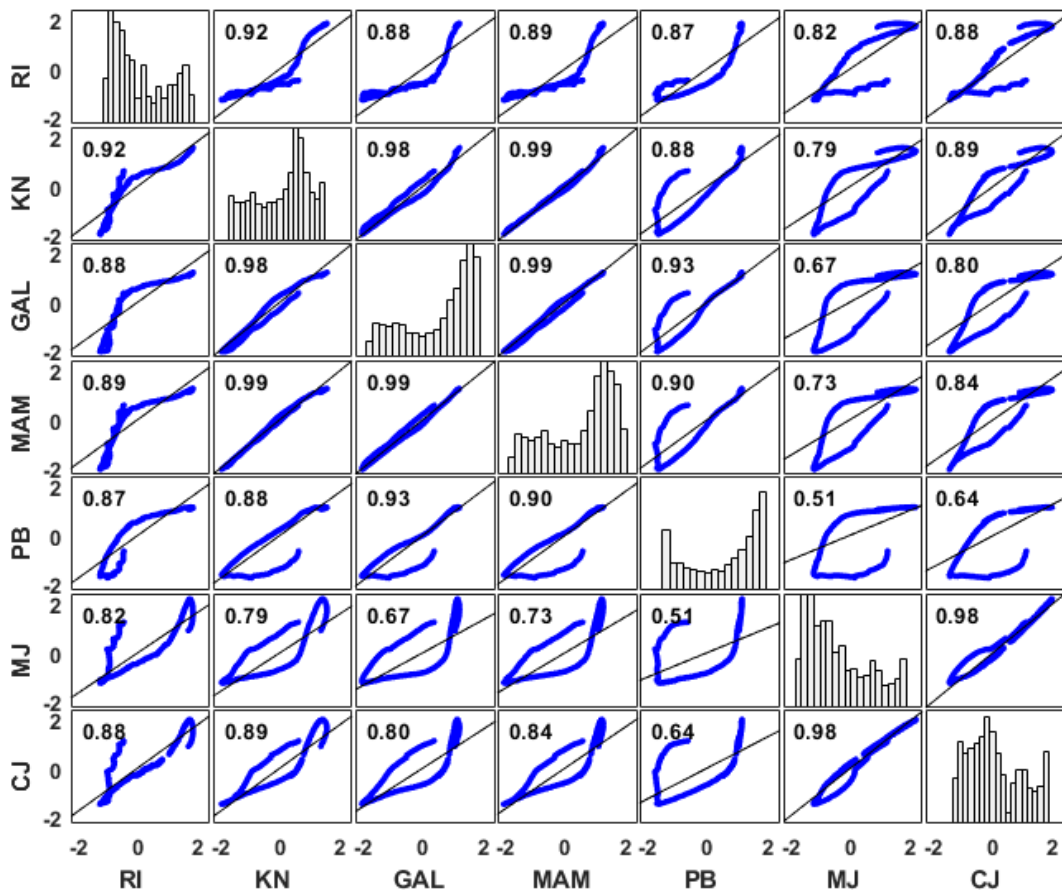
Slika 2.34 Matrica korelacija između razina vode u Ričicama (RI), Knezovića jezeru (KN), Galipovcu (GAL), Mamića jezeru (MAM), Prološkom blatu (PB), Modrom jezeru (MJ) i Crvenom jezeru (CJ)
