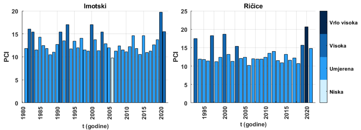
Slika 2.11 Indeks koncentracije oborina (PCI) na godišnjoj razini na postajama Imotski i Ričice
