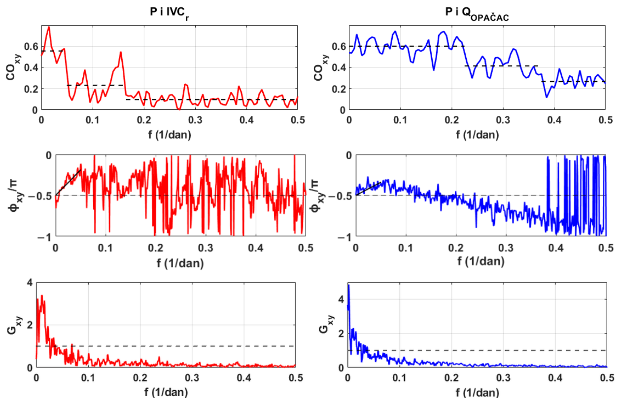
Slika 2.32 Funkcija koherencije CO_{xy} , faza funkcija \Phi_{xy} i funkcija prigušenja ili pojačanja G_{xy} oborina s integralnim promjenama volumena u Crvenom jezeru i protocima na Opačcu
