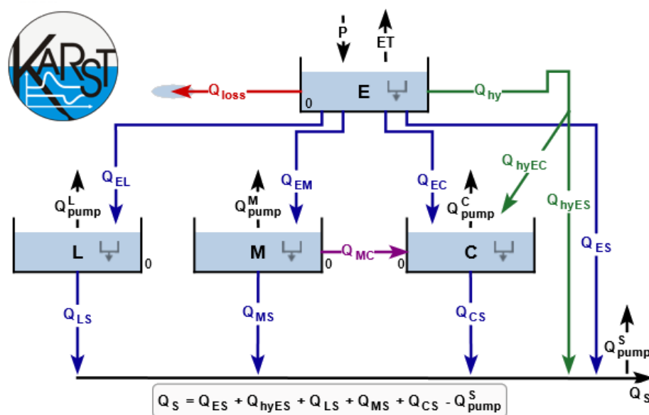
Slika 3.1 Struktura modela u KARSTMODU pri aktivaciji svih dostupnih odjeljaka
