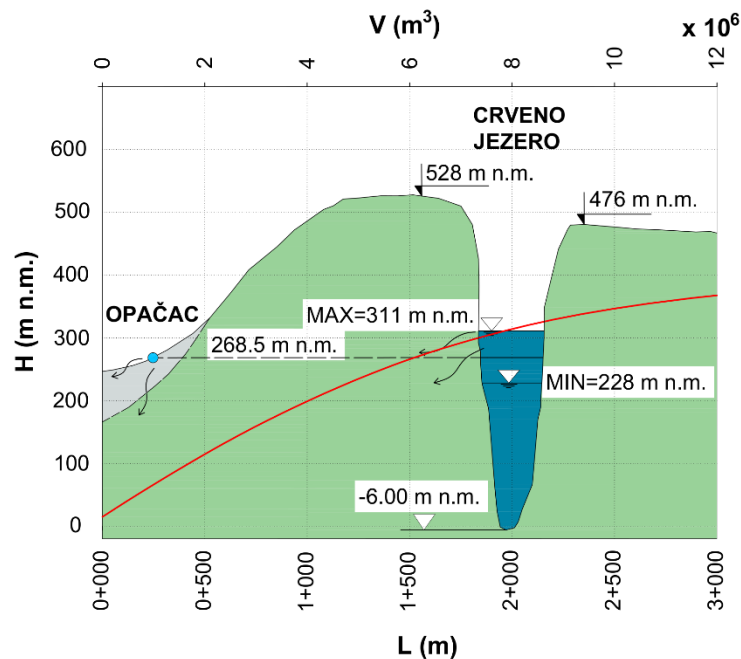
Slika 1.7 Krivulja volumena Crvenog jezera u funkciji razine vode, uz prikaz poprečnog presjeka Crvenog jezera i izvora Opačac s naznačenim zabilježenim minimumom i maksimumom u Crvenom jezeru
